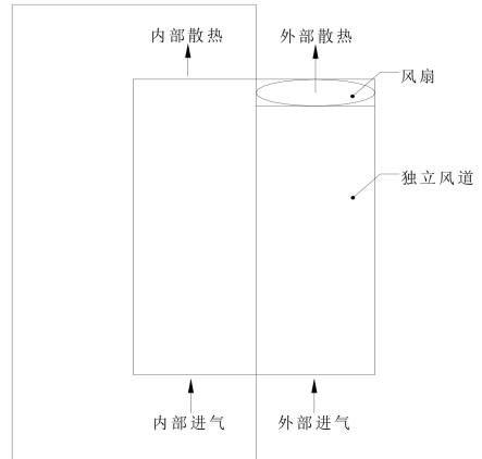
图 2- 5 透壁安装方式
