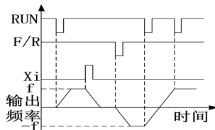
(b) F04.19=0, F00.03=2 正/反转运行逻辑
