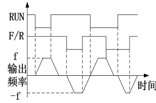
(d) F04.19=0, F00.03=1 运行正/反转逻辑
