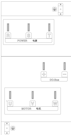
(e) 380V 250-400kW、660V 315-450kW 主功率端子
