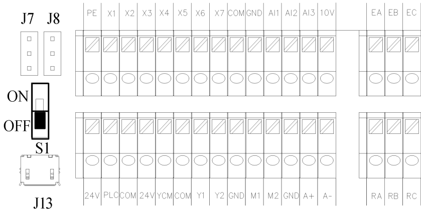
图 3-6 控制回路端子排列
