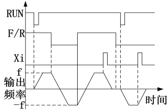
(d) F04.19=0, F00.03=3 正/反转运行逻辑
