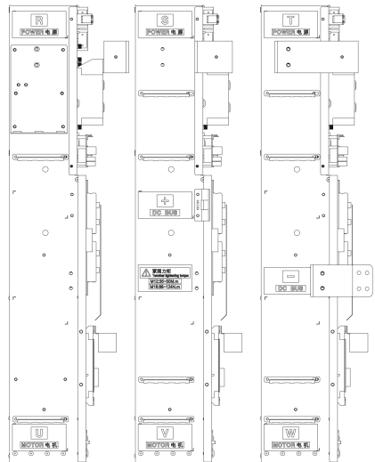
(f) 450-560kW 主功率端子
