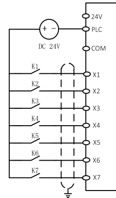
图 3-7 多功能输入端子接线图
