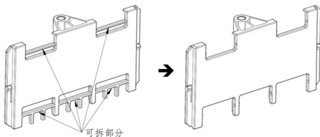
图 3-3 过线板
